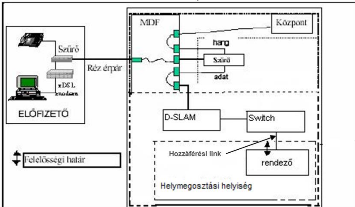
Közele bitfolyam hozzáférés réz érpáras hálózaton, helymegosztás esetén
